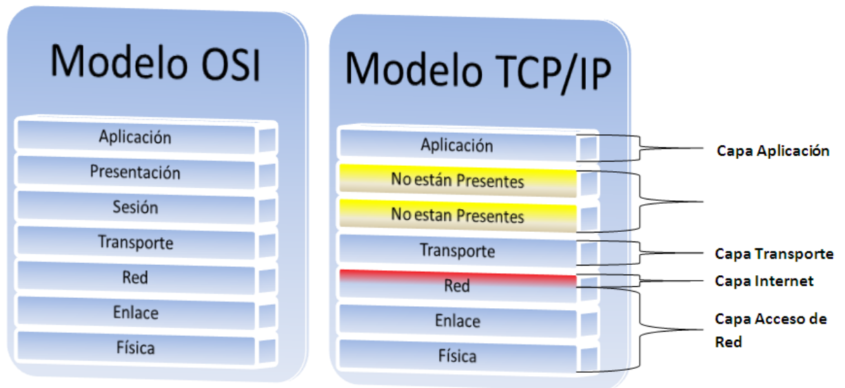
Figura 7. Modelo OSI vs TCP/IP
