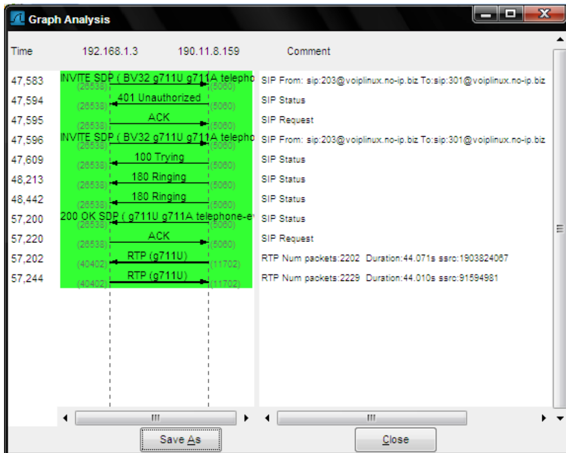
Figura 94 Gráfica de la llamada VoIP Fuente: Captura de paquetes con Wireshark
