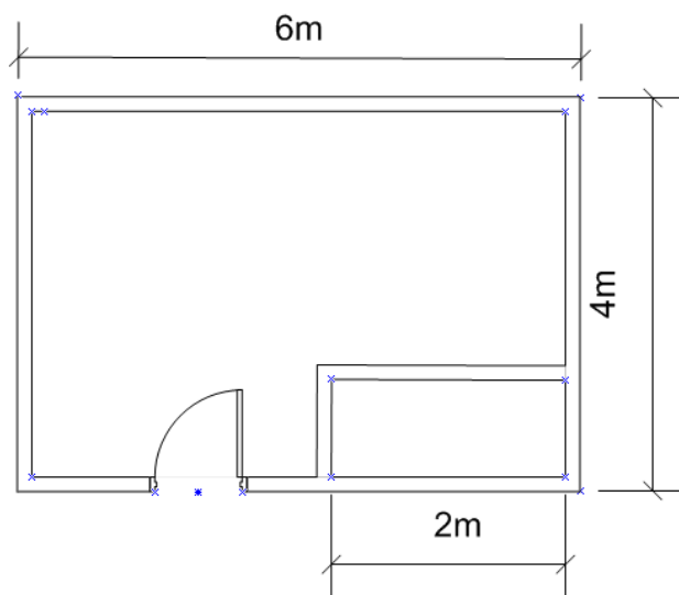
Figura 110 Plano Oficina Tena Elaborado por: Cristian Puga
