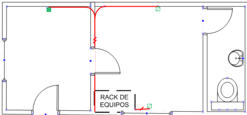
Figura 113 Cableado de la Oficina Lago Agrio Elaborado por: Cristian Puga
