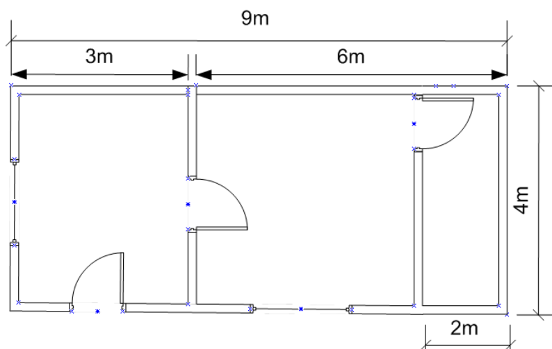
Figura 109 Plano Oficina Lago Agrio
