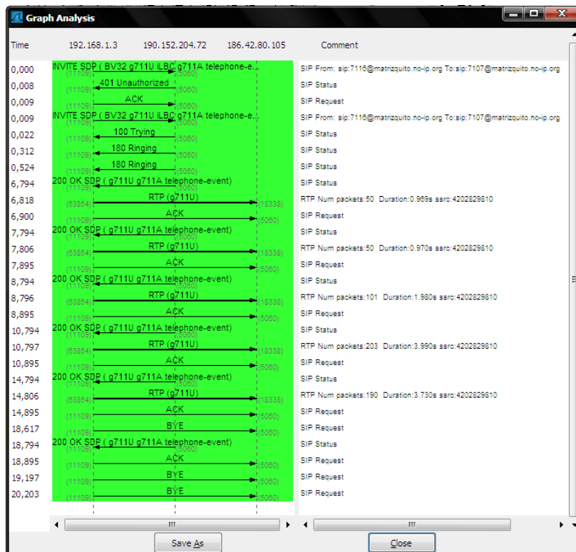
Figura 91 Gráfico de Transmisión de Paquetes
