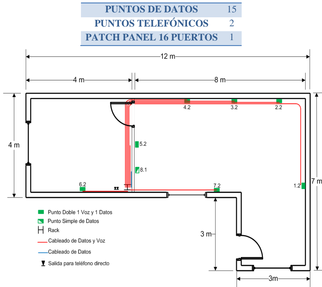
Figura 18 Cableado Estructurado Oficina Quito
