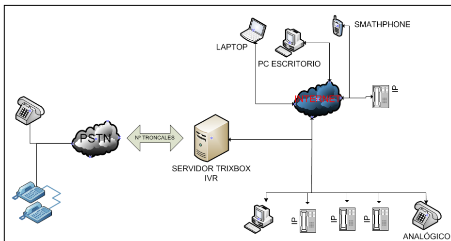
Figura 51 Esquema del IVR a implementarse
