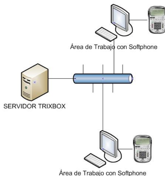
Figura 87 Servidor VoIP y 2 extensiones
