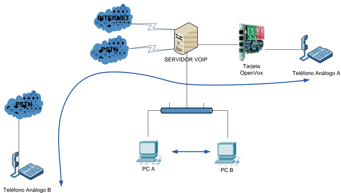
Figura 99 Esquema del Proceso de Llamada
