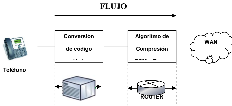
Figura 13. PBX y Router en red VoIP
