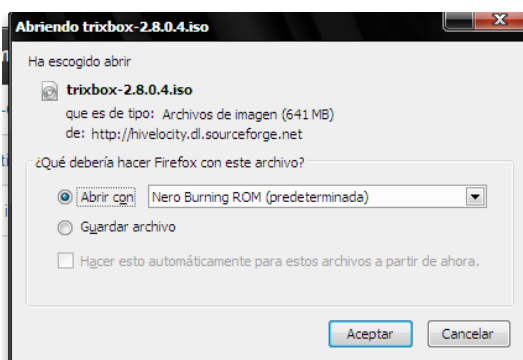
Figura 33 Descargando TRIXBOX
