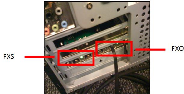
Figura 16. Fotografía de equipo Real
