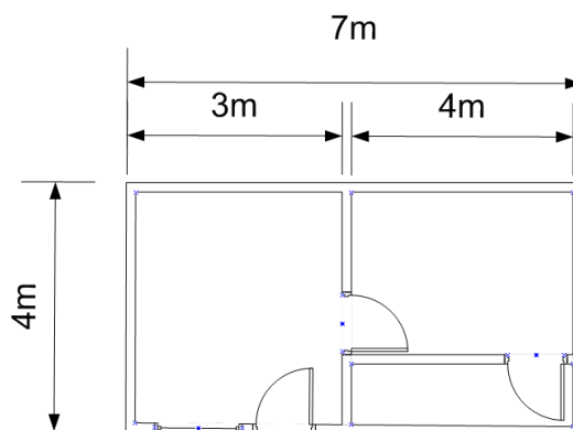
Figura 112 Plano Oficina Puyo Elaborado por: Cristian Puga
