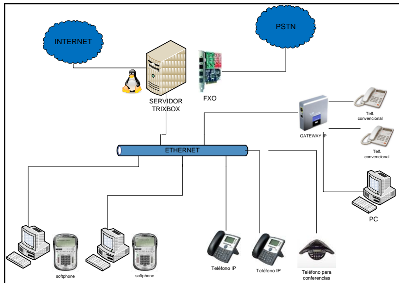
Figura 21 Diagrama de la red LAN
