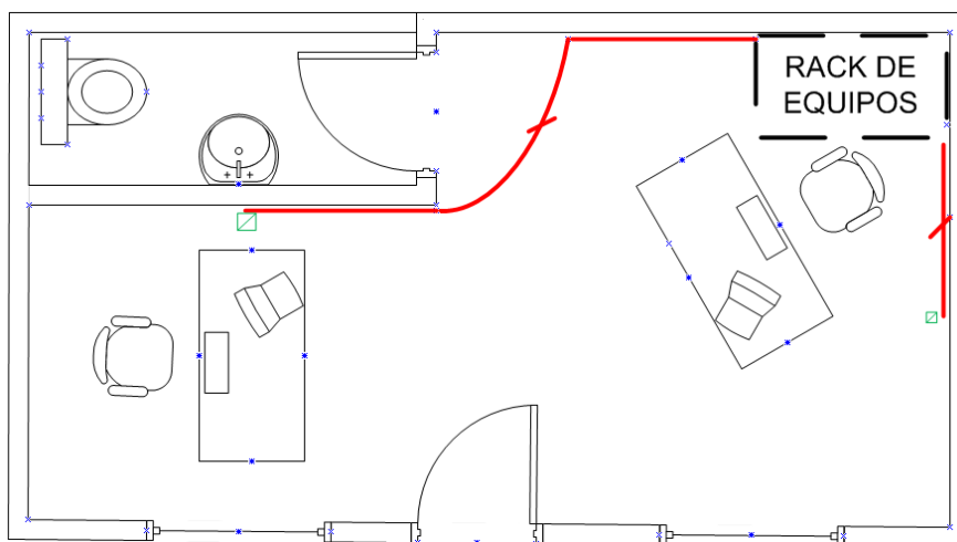
Figura 114 Cableado de Oficina Pto. Francisco de Orellana Elaborado por: Cristian Puga
