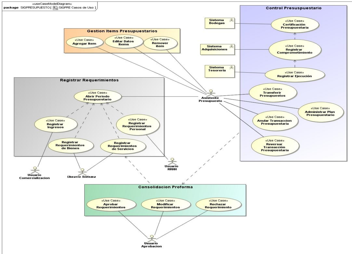
Figura 4 Diagrama de Casos de Uso del sistema de Gestión Presupuestaria
