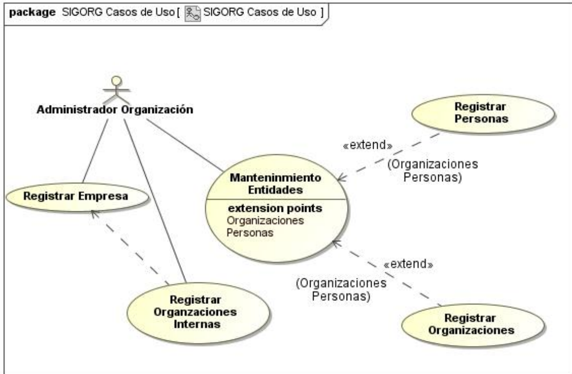
Figura 1 Casos de Uso modulo Organizacional
