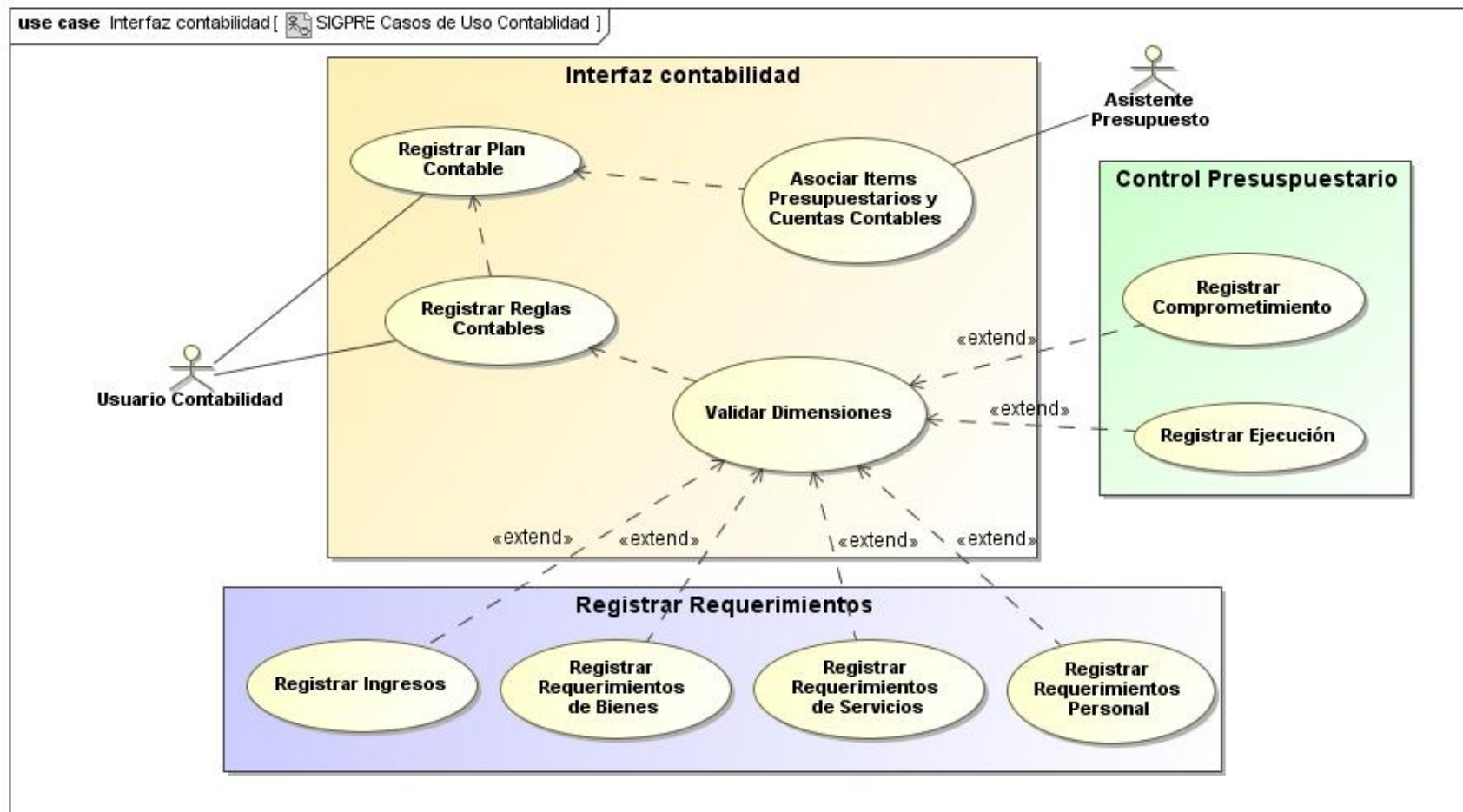
Figura 5 Modelo de Casos de Uso Interfaz Contable
