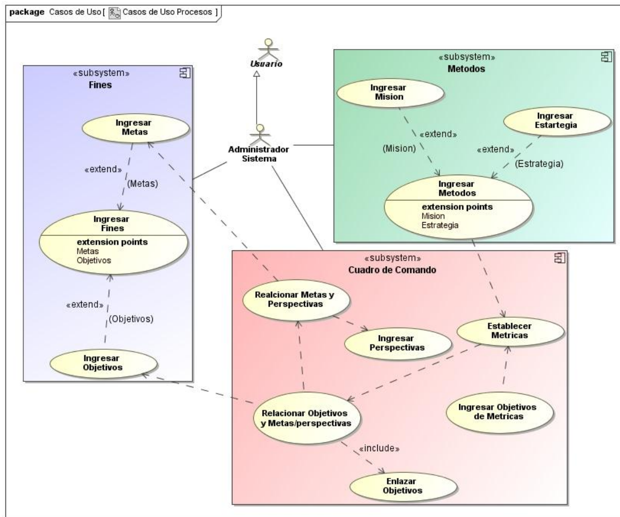
Figura 3 Modelo de Casos de Uso para planificación estratégica
