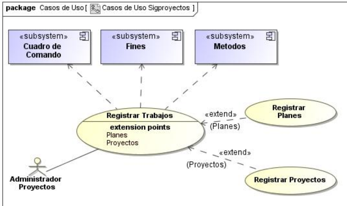
Figura 2 Casos de Uso del módulo de proyectos
