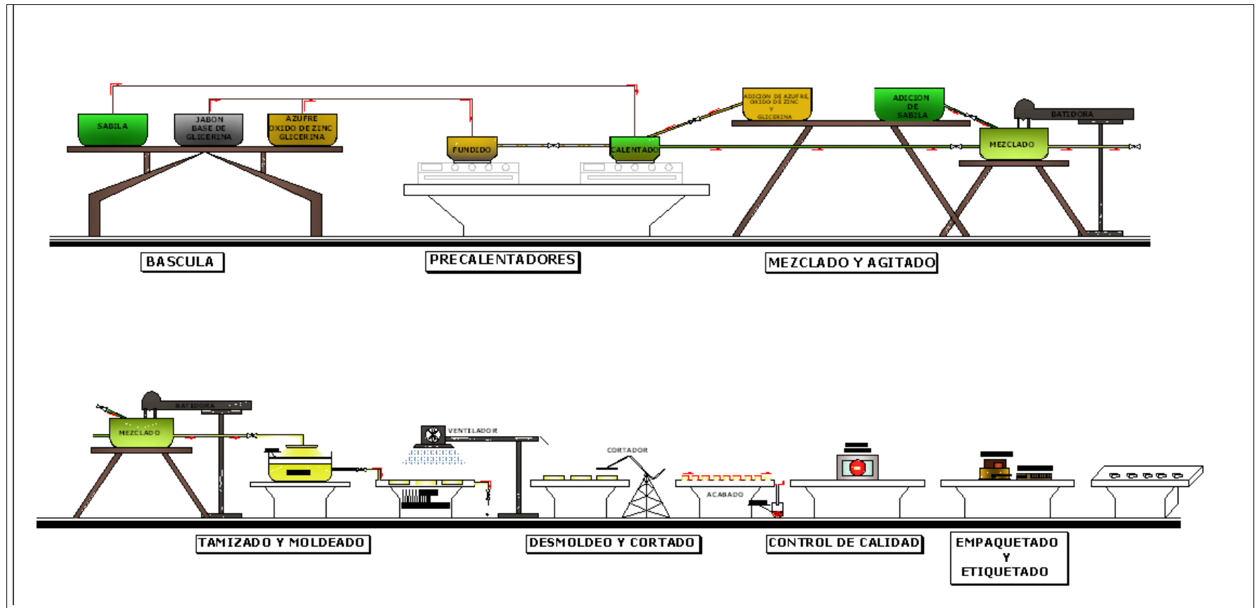
Anexo 5: Diagrama ingenieril para la elaboración de jabón de tocador sulfurado, antiséptico y humectante.
