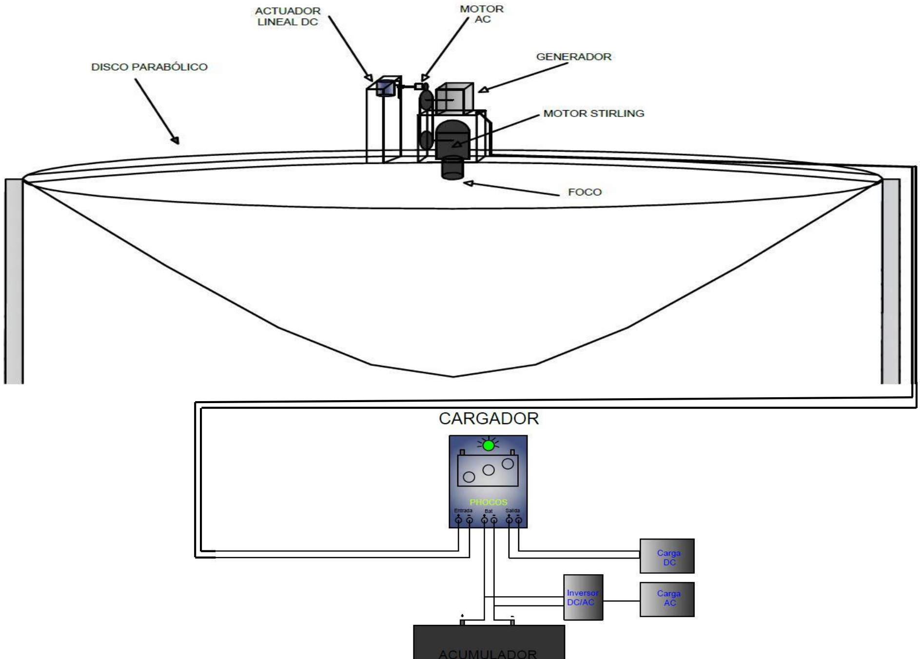
ANEXO 9: Diagrama general del sistema de generación termo solar disco-Stirling.
