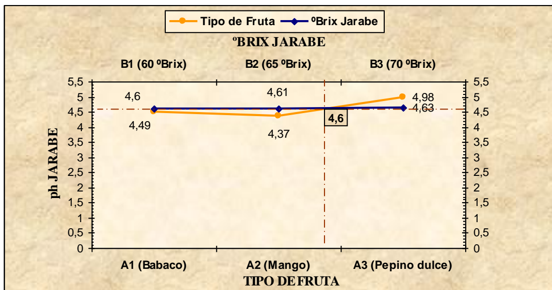
Gráfico 3: Interacción de los factores: A (Frutas) y B (Sólidos solubles en el jarabe) para la variable pH del jarabe en la etapa media de la deshidratación osmótica
