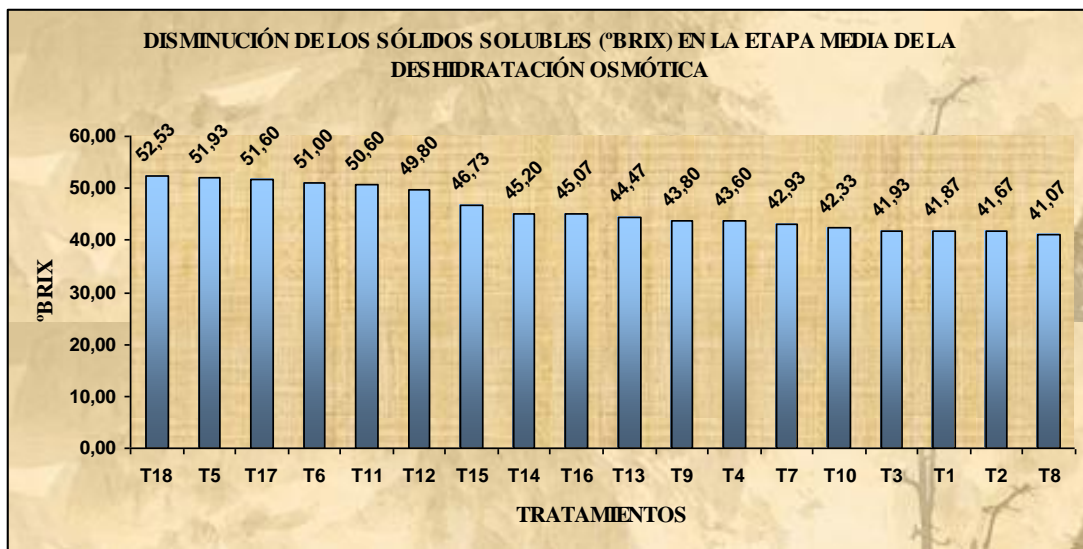
Gráfico 8: Disminución de sólidos solubles en la etapa media de la deshidratación osmótica
