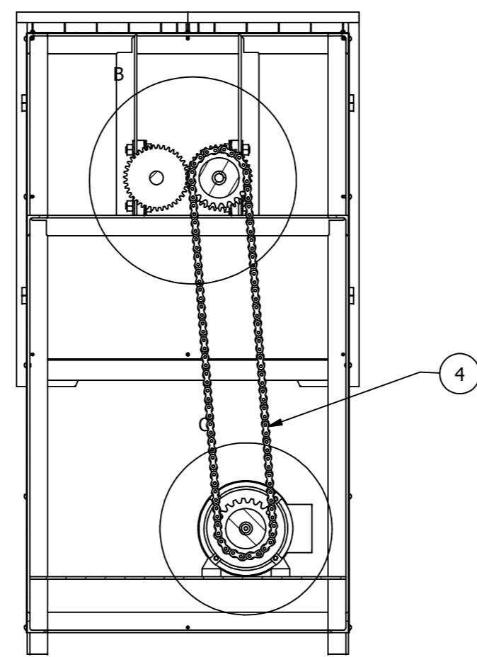
A-A (1 : 10)
