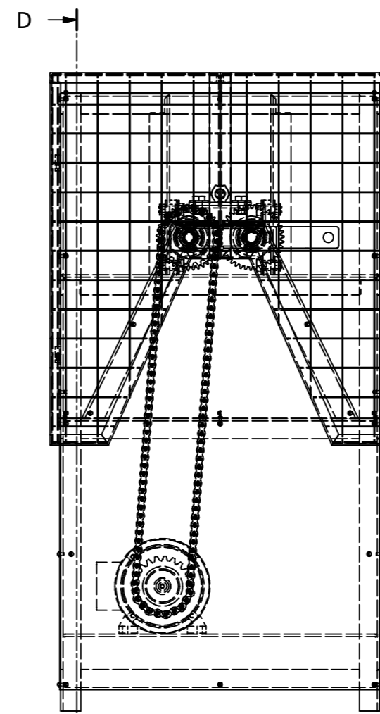
E (1 : 10)
