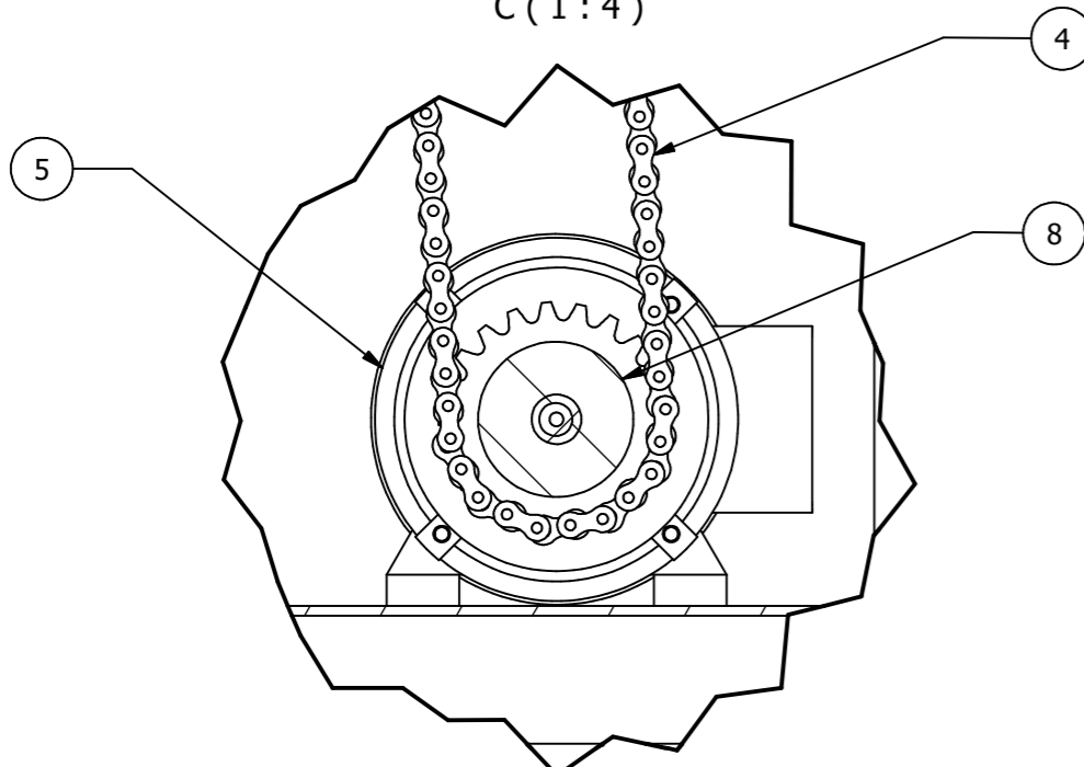
C (1 : 4)
