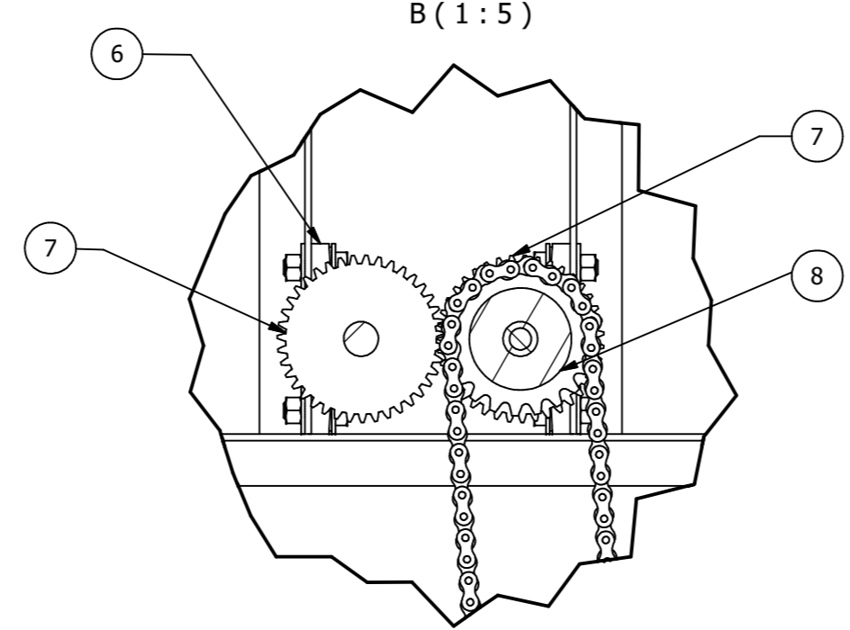
B (1 : 5)
